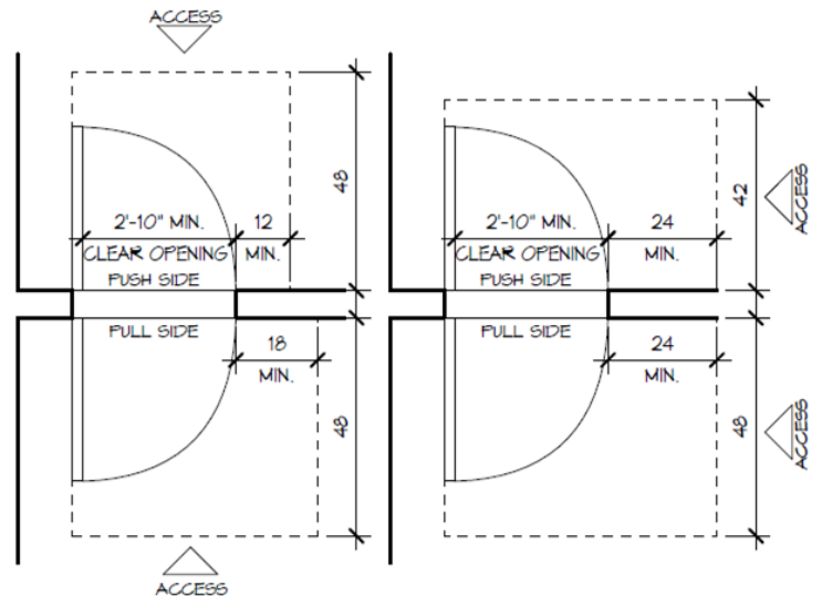
Door Clearances
